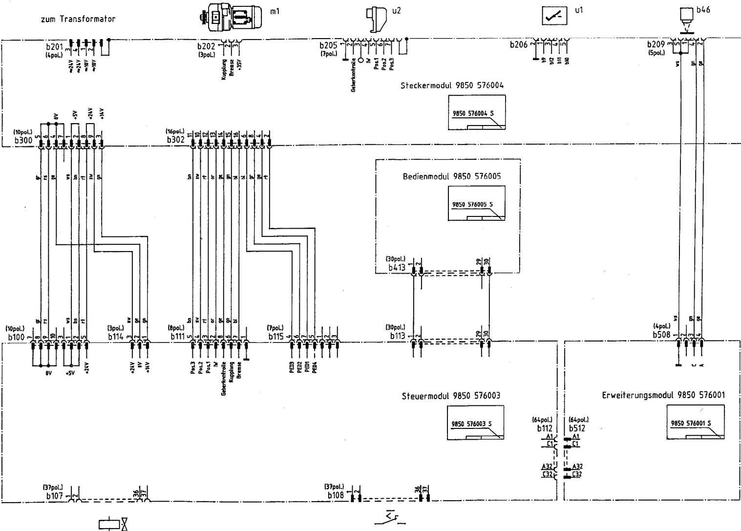
Bauschaltplan 9890 576001 B
