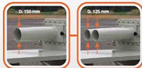
Односопловая форсунка
