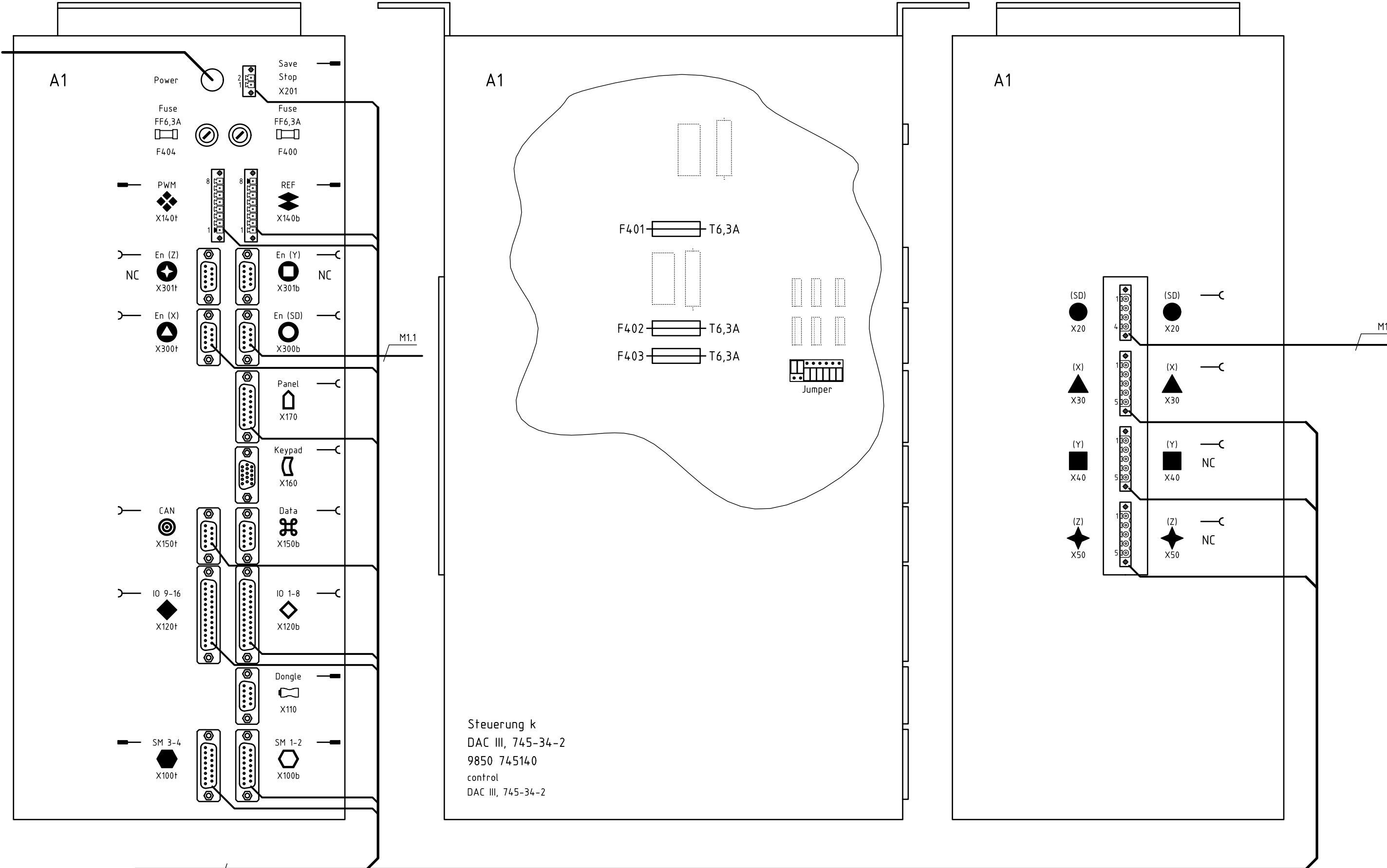
Kabelbaum 9870 745165
