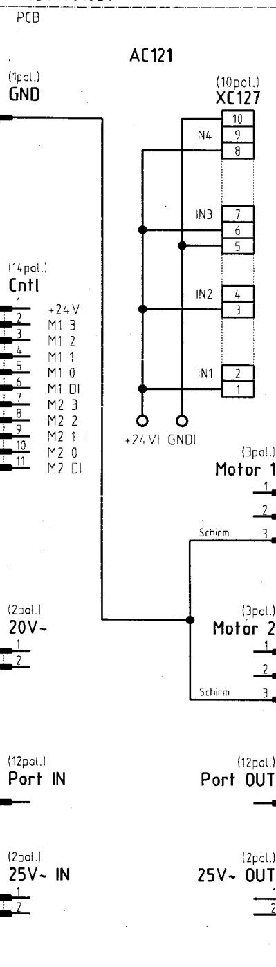
Leiterplatte k 9850 001051
