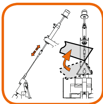
Точка выворачивания воротника Reversing collar point
